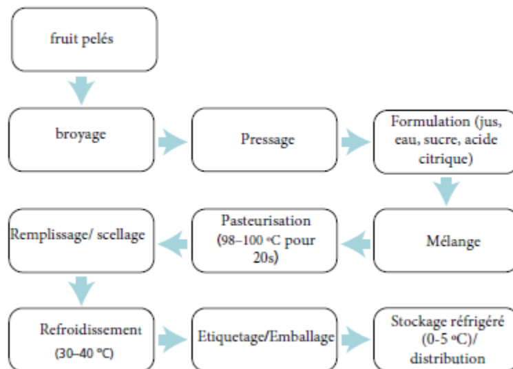
Figure 7 Processus de fabrication du jus de figues de Barbarie
